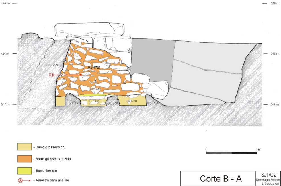
Fig. 35. Mosteiro de São João de Tarouca – corte estratigráfico B-A da fossa sineira Fonte: Desenho de Luís Sebastian e Hugo Pereira
