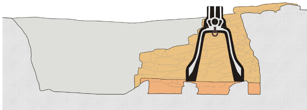
Fig. 40. Mosteiro de São João de Tarouca – reconstituição da fossa sineira (corte transversal)
