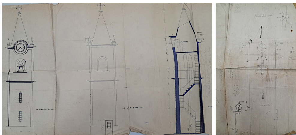
Fig. 3. Alçado do projeto inicial para a torre do relógio de Corte do Pinto
