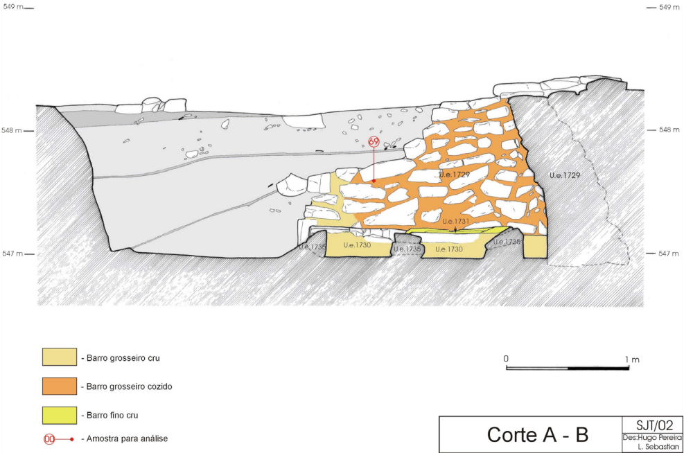
Fig. 36. Mosteiro de São João de Tarouca – corte estratigráfico A-B da fossa sineira Fonte: Desenho de Luís Sebastian e Hugo Pereira
