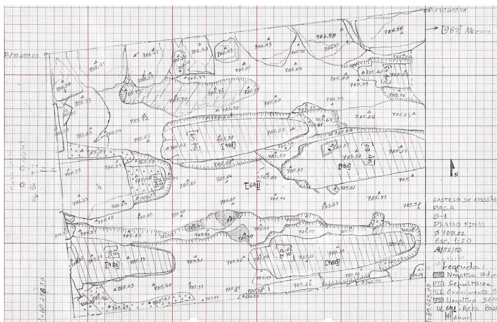
Fig. 27. Igreja de São Salvador de Ansiães – planta geral da fossa sineira
