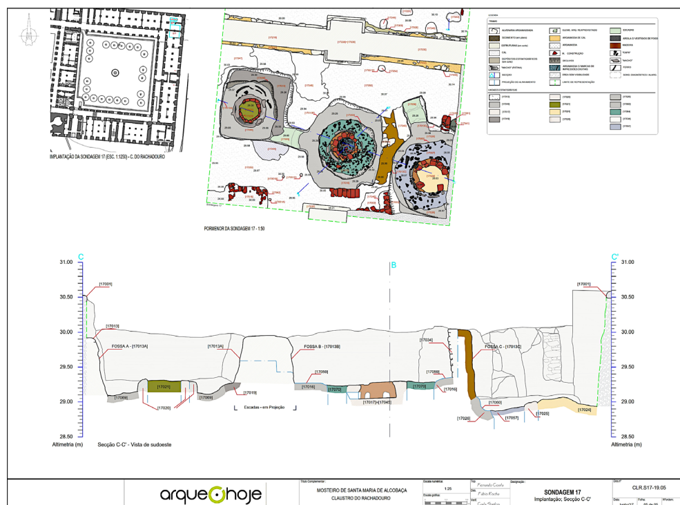
Fig. 50. Mosteiro de Santa Maria de Alcobaça – planta geral e secção das três fossas sineiras
