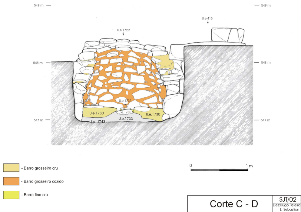
Fig. 37. Mosteiro de São João de Tarouca – corte estratigráfico C-D da fossa sineira Fonte: Desenho de Luís Sebastian e Hugo Pereira
